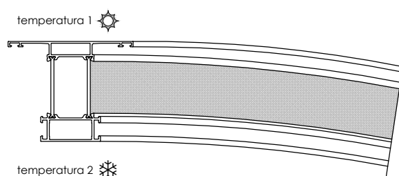
Dilatazione in caso di ELEMENTI VINCOLATI
